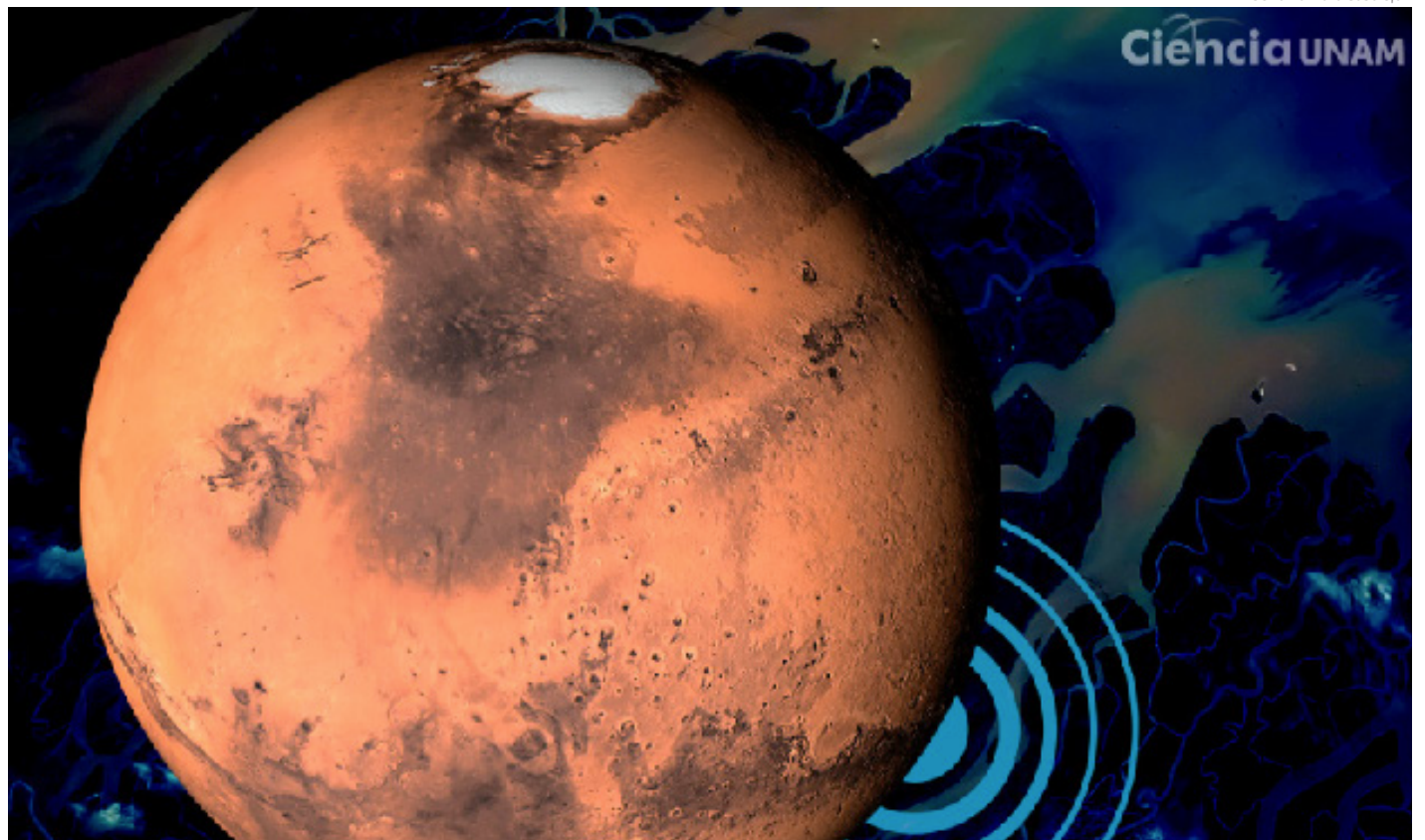
El análisis indica que los depósitos de agua se encuentran a profundidades de entre 10 y 20 km por debajo de la corteza marciana.
