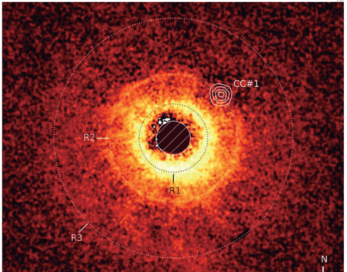
Imagen del disco alrededor de la estrella TWA 7 registrada con el instrumento SPHERE del Very Large Telescope de la ESO. La imagen capturada con el instrumento MIRI del JWST se superpone. Podemos ver claramente el área vacía alrededor de TWA 7 B en el anillo R2.
