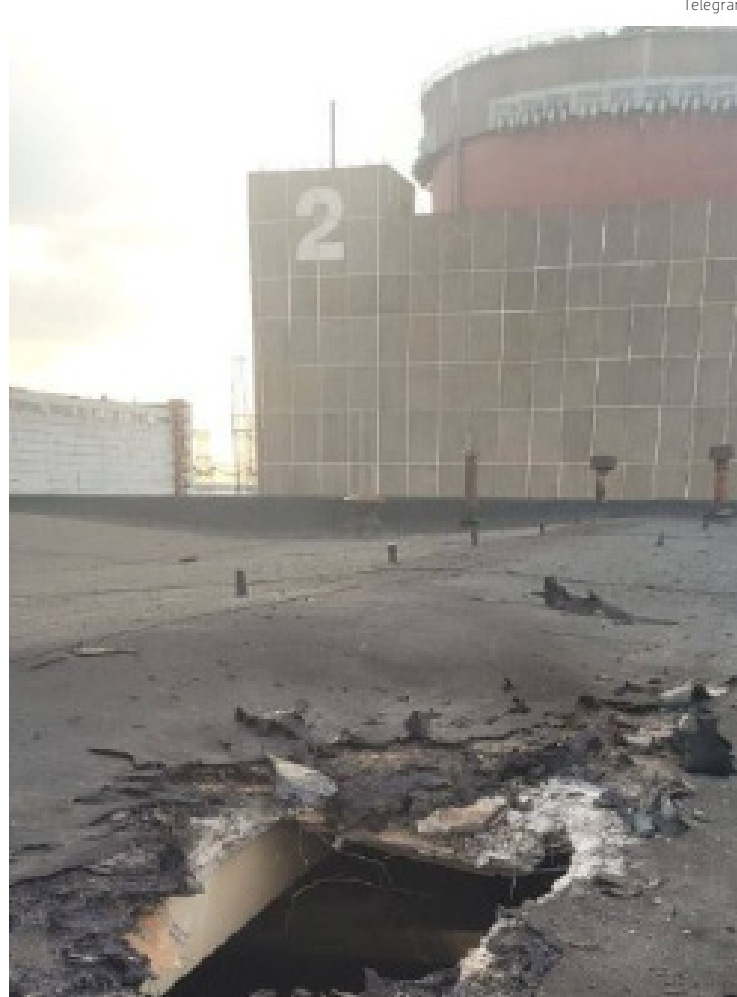
Boquete en el techo de uno de los reactores de la central de Zaporíyia.
