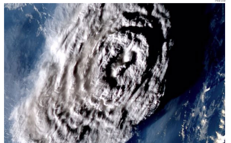
La pluma del volcán Tonga.
