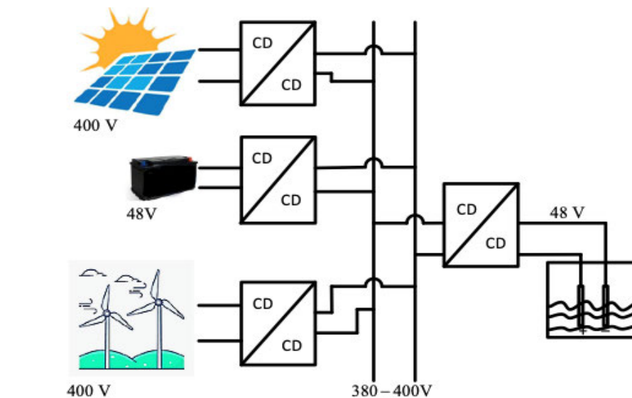
Microrred alimentando a un electrolizador.
